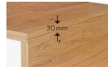
Profil 30 Stil Block Abdeckung für ein vollendetes Design (auf Gehrung gearbeitet, Radius 3 mm).
